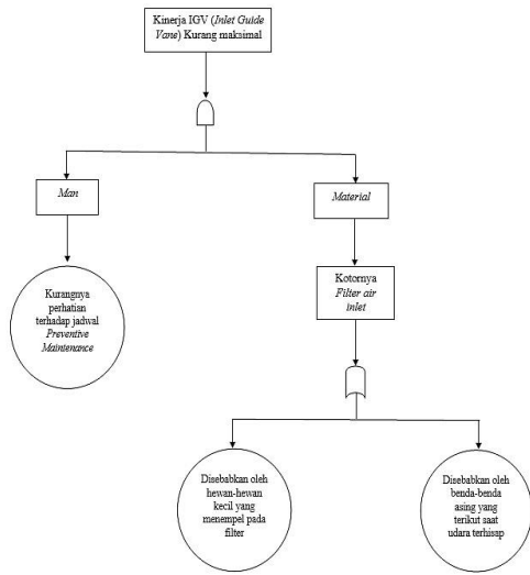
Gambar 3. Fault tree kurang maksimalnya kinerja Inlet Guide Vane ((IGV)
