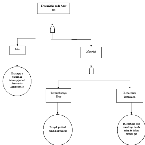
Gambar 4. Fault tree Unreadable pada filter gas
