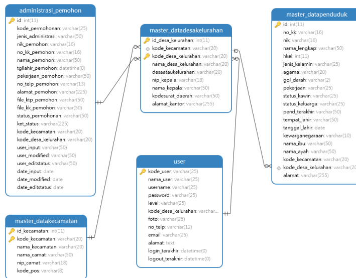
Gambar 4. Desain Relasi Database
