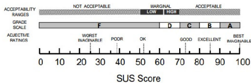
Gambar 11. Skor SUS
