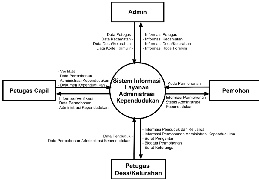
Gambar 2. Diagram Konteks
