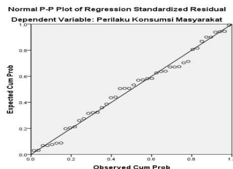
Gambar 1. Hasil Uji Normalitas dengan P-P Plot
