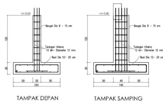
Gambar 5 Pondasi Tapak (Sumber: Google, 2022)
