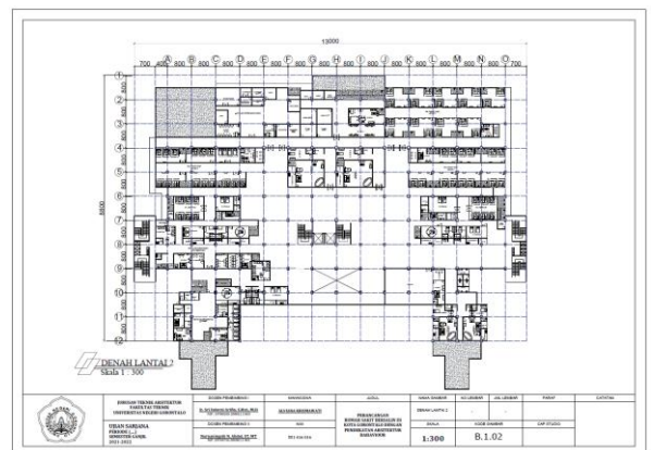
Gambar 13. Denah Lantai 2 (Sumber: Hasil Analisis, 2021)
