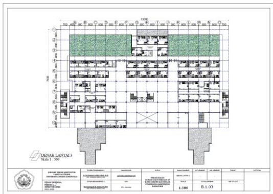
Gambar 14. Denah Lantai 3 (Sumber: Hasil Analisis, 2021)
