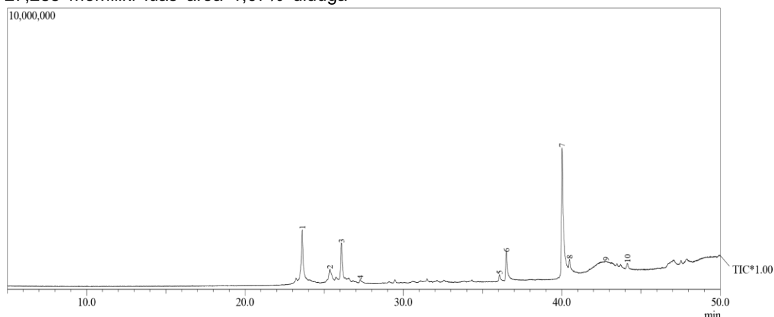
Gambar 1. Kromatogram (KG) Sampel Metil ester (Minyak Biji Kelor Kering)
