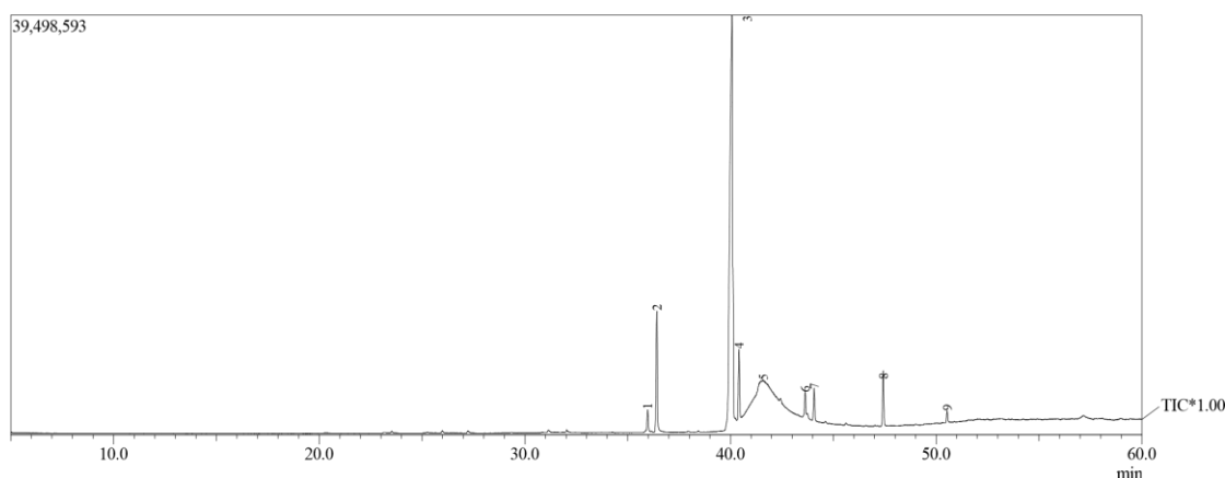
Gambar 2. Kromatogram (KG) Sampel Metil ester (Minyak Biji Kelor Basah)
