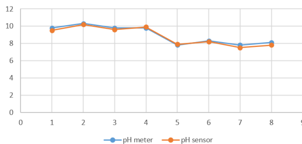
Gambar 5 Grafik perbandingan nilai rata-rata pH meter dan pH sensor
