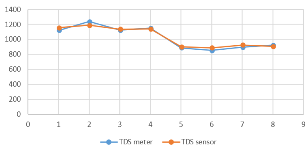
Gambar 4 Grafik perbandingan nilai rata-rata TDS meter dan TDS sensor
