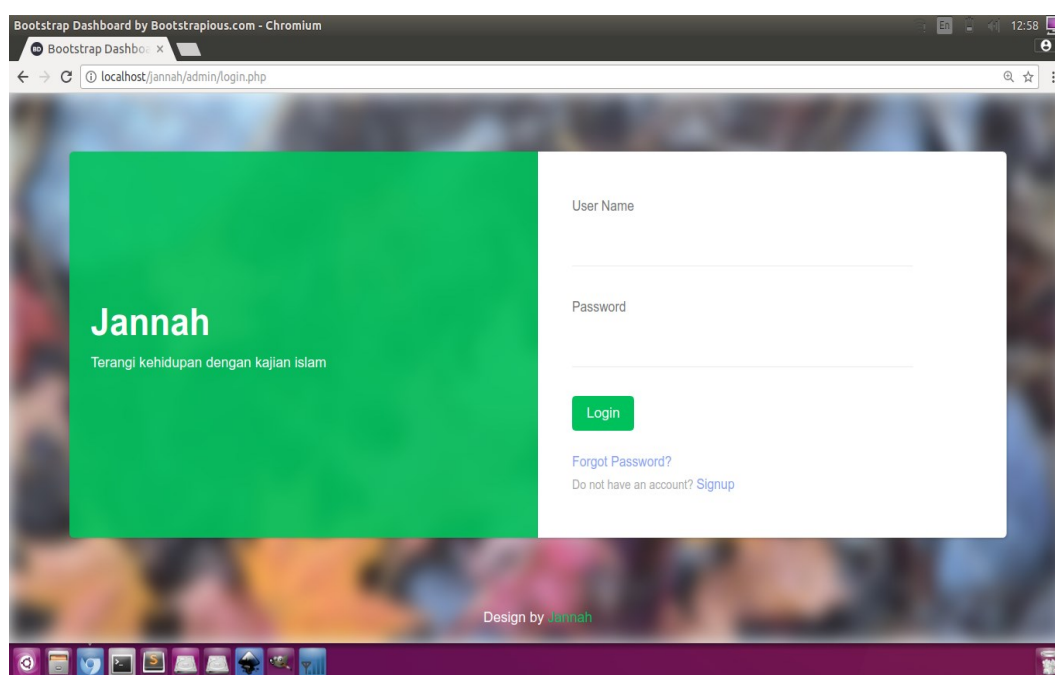
Gambar 4. Halaman login
