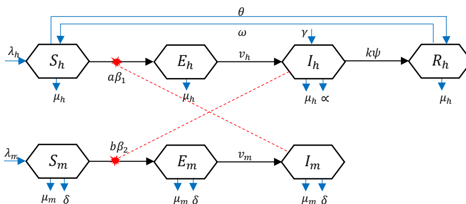
Gambar 1. Diagram kompartemen transmisi penyakit malaria dengan vaksinasi dan pengasapan
