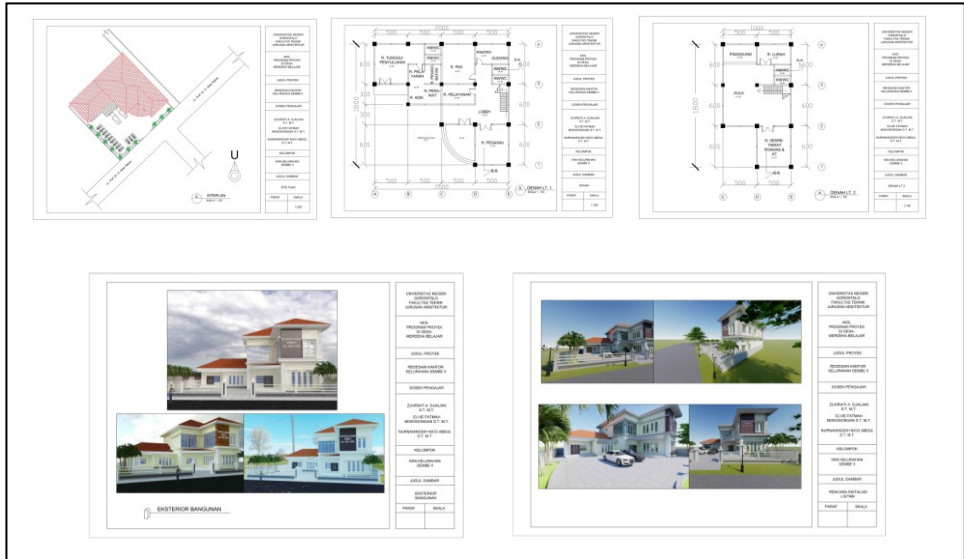
Gambar 11. Denah dan Perspektif Kantor Kelurahan Dulomo Utara
